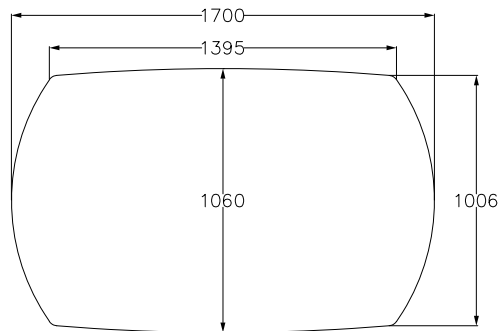
Pianta — Chiuso
