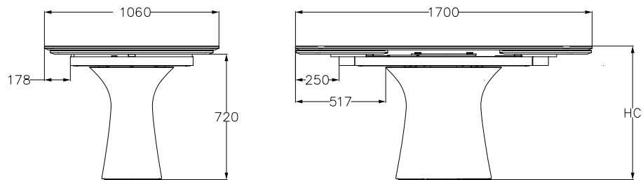
Vista Laterale—Chiuso
