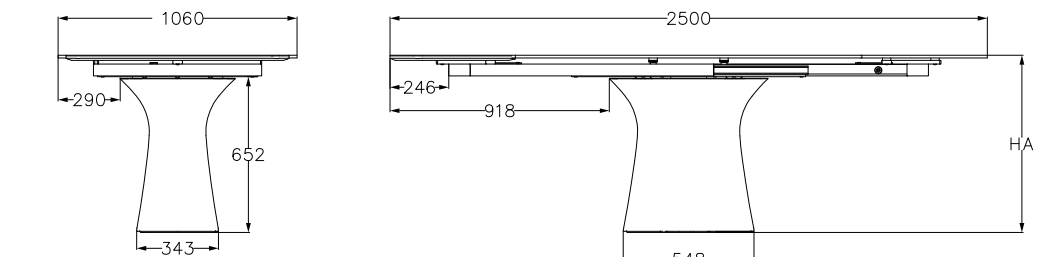
Vista Laterale—Aperto
