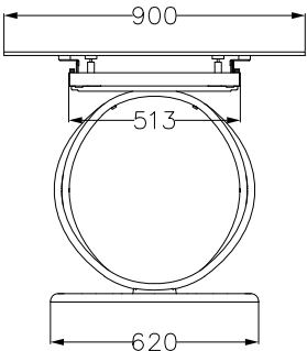
Vista Laterale
