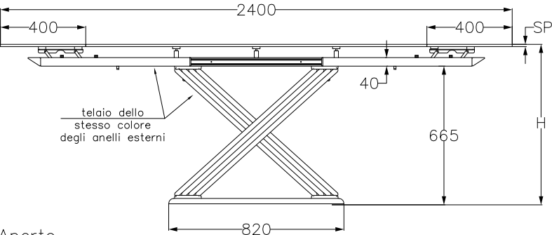
Aperto
